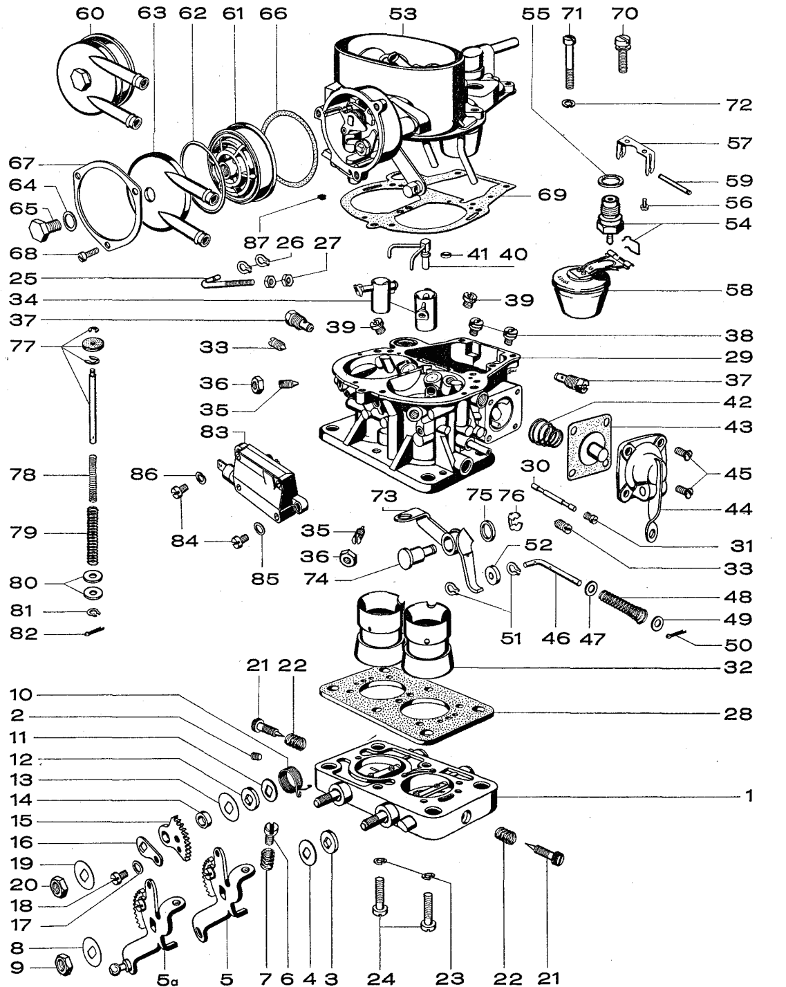
Bild 78 Solex-Vergaser 32 DDIST, Montagebild
