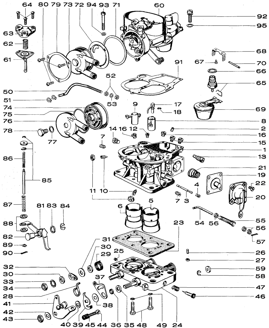
Bild 75a Solex-Vergaser Typ 32 TDID, Montagebild
